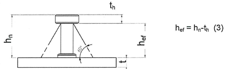
Abb. 3: Kurzer Kopfbolzen, wenn der theoretische Ausbruchkegel im Winkel von \sim 60^\circ auf die Stahlplatte trifft, oder t \geq 0,2 h_n
