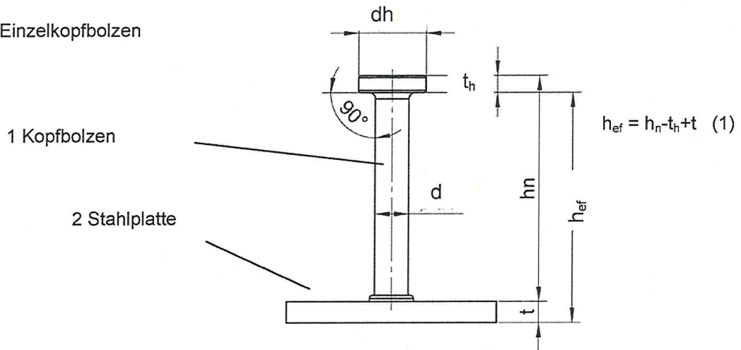
Abb. 2: Zusammengesetzte Kopfbolzen
